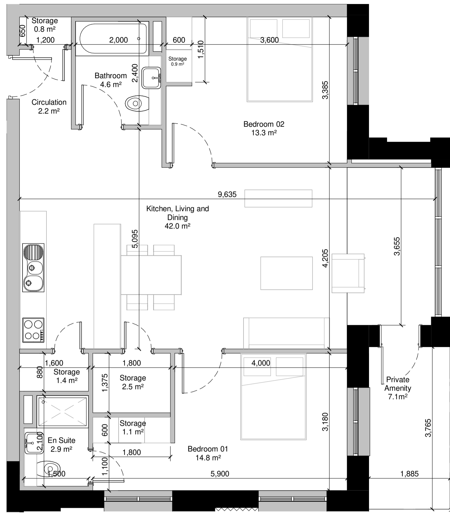
1 Type B2_2.7 - 2B4P 1 : 50
